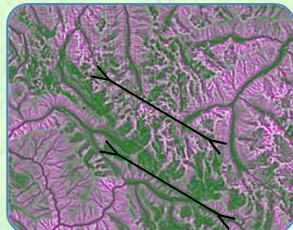
Seismic zonation
